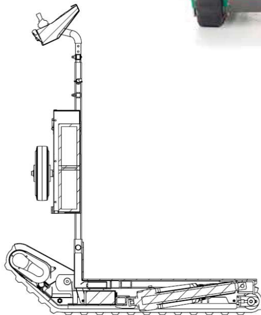
Sezione A-A
